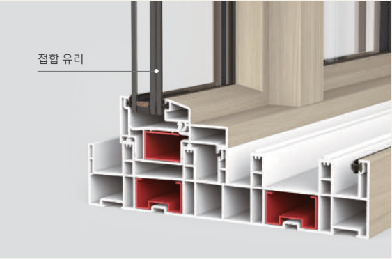
안전한 접합 유리 두 장의 유리 사이에 PVB 접합 필름을 삽입 후 고압으로 압착한 유리 입니다. 파손이 되더라도 조각이 떨어져 나가지 않아 안전합니다. *난간대가 없는 경우 하부 접합 유리를 필수 적용하여 안정성을 높입니다.
